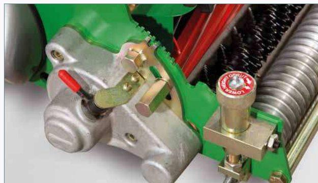
Innesto della trasmissione del groomer facile da azionare
