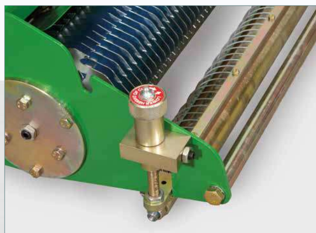
Regolazione semplice dell'altezza di funzionamento senza l'utilizzo di utensili
