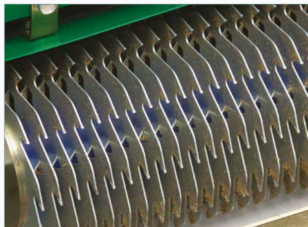
Il verti-cutter definitivo con lame con punte al tungsteno
