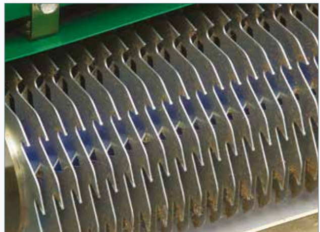
Lo sfeltratore verticale a lame definitivo con lame con punte al tungsteno
