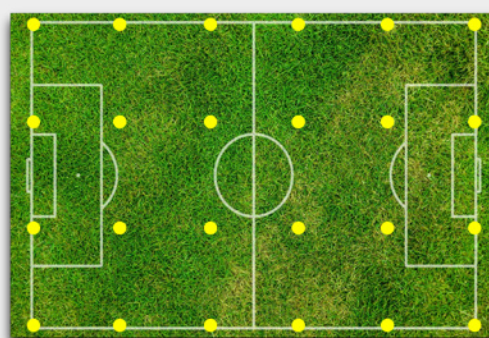
ESEMPIO SU SCHEMA STANDARD A 24 IRRIGATORI
